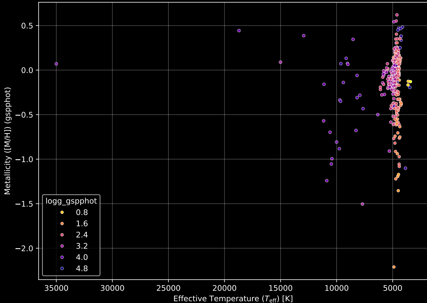
APOGEE DR17 Field: [060-08] Stellar Population Parameters (n= 458)
